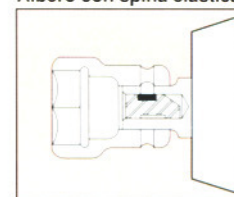
Albero con spina elastica
